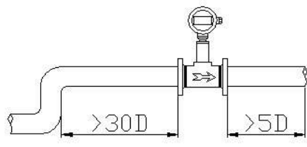
上游有两个90度直角弯头 流量计前直管段保证大于30D
