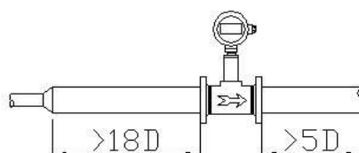
上游有扩径大小头 流量计前直管段保证大于18D
