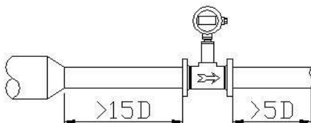
上游有缩径大小头 流量计前直管段保证大于15D
