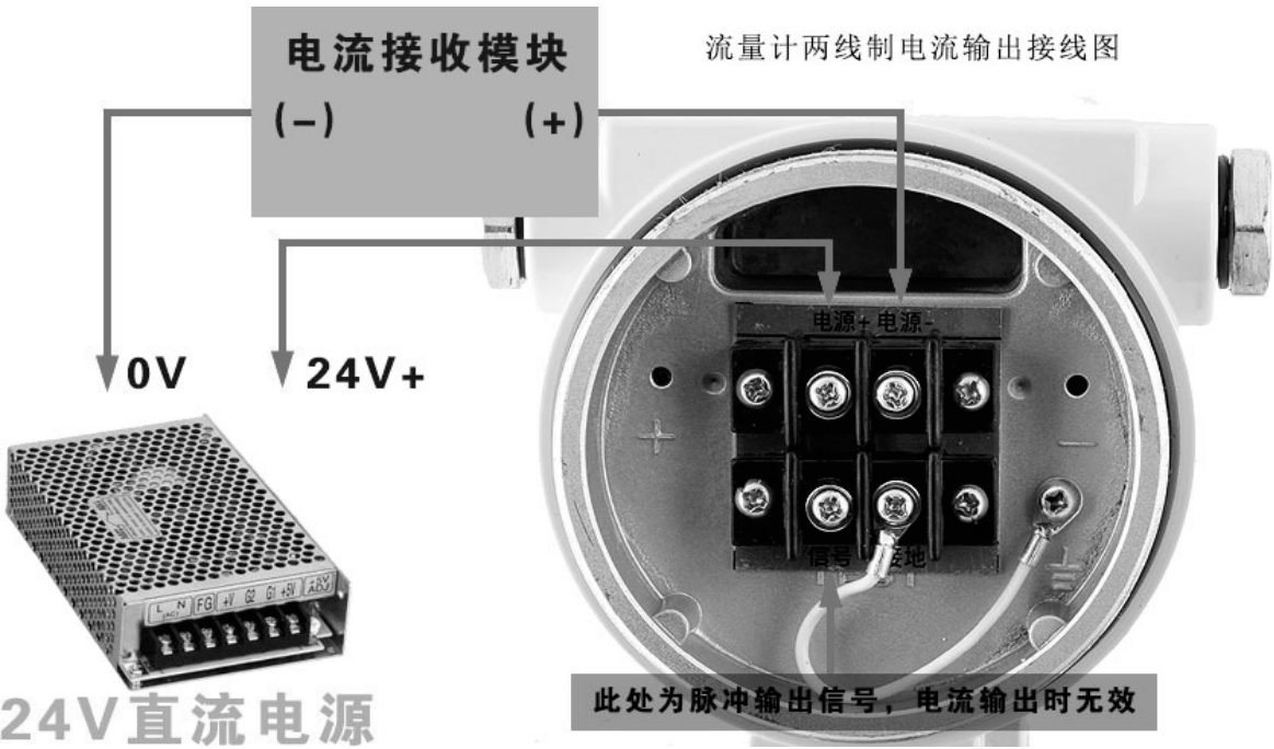
4~20mA 电流输出接线示意图:
